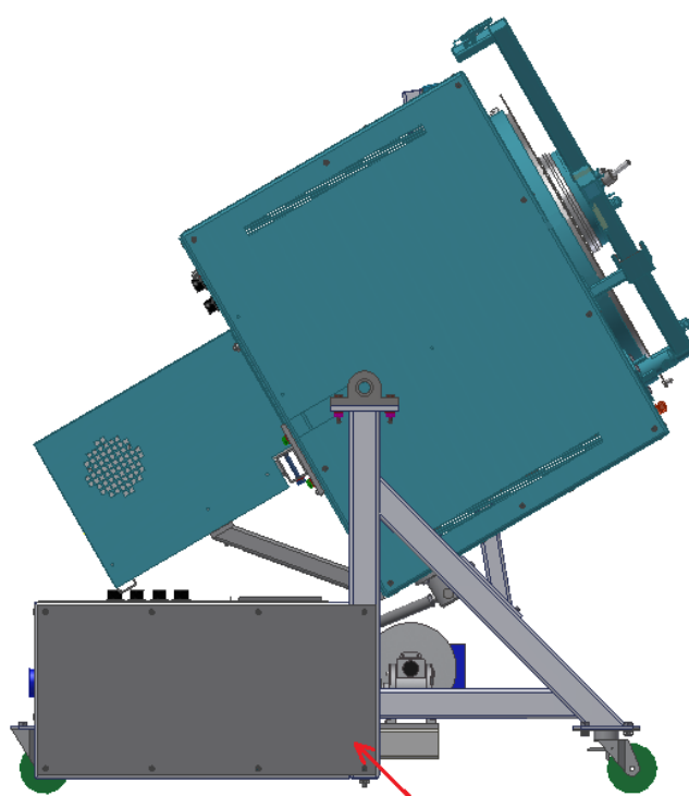
Рисунок 30 - Кожух блока управления, закрывающий трапецидальный винт
