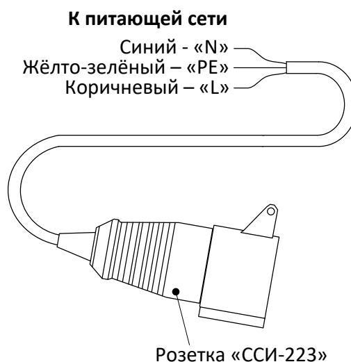
Рисунок 3 - Соединитель питания
