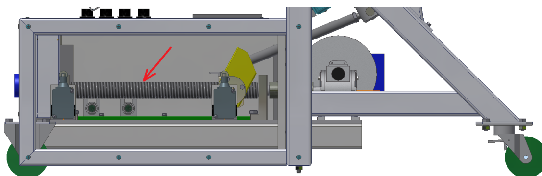
Рисунок 31 - Трапецидальный винт
