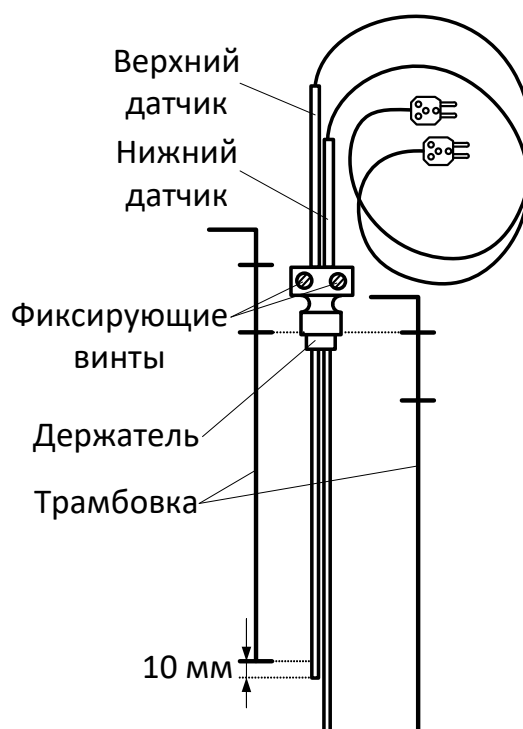
Рисунок 12 – Регулирование датчиков температуры реактора
