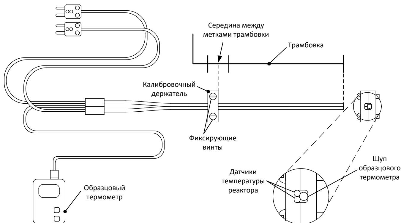
Рисунок 16 – Установка датчиков в калибровочный держатель
