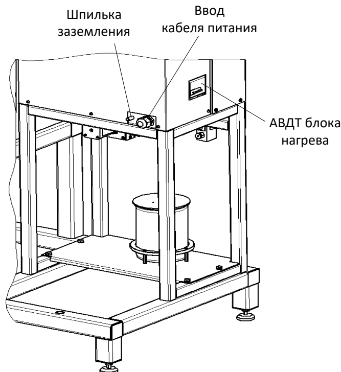
Рисунок 2 – Питание устройства
