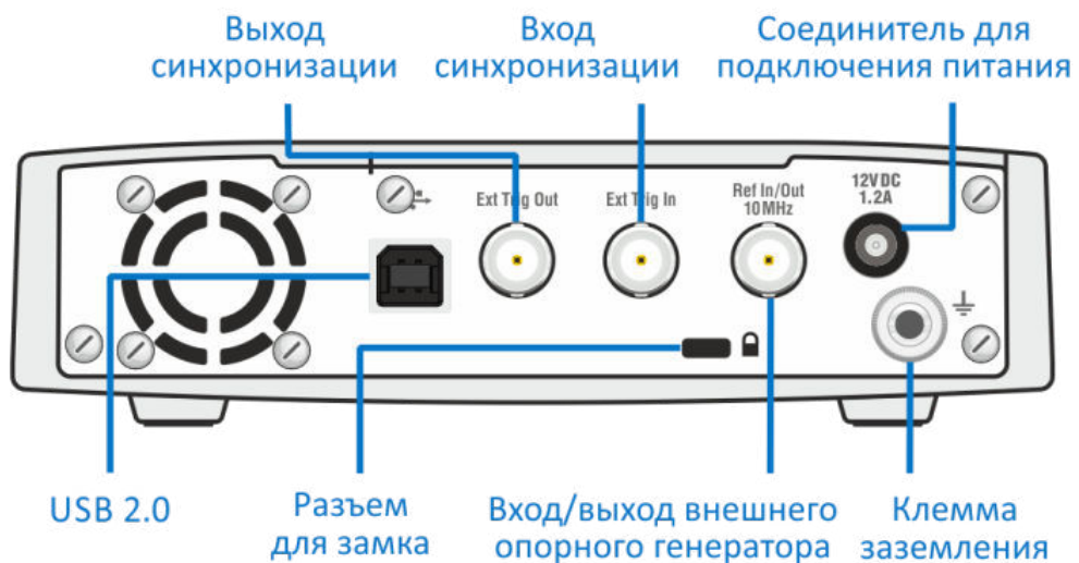
Рисунок 4.6 Задняя панель
