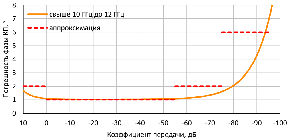
Погрешность измерений фазы коэффициента передачи согласованных устройств анализаторов S50180 (при уровне выходной мощности 0 дБм и полосе фильтра промежуточной частоты 1 Гц)
