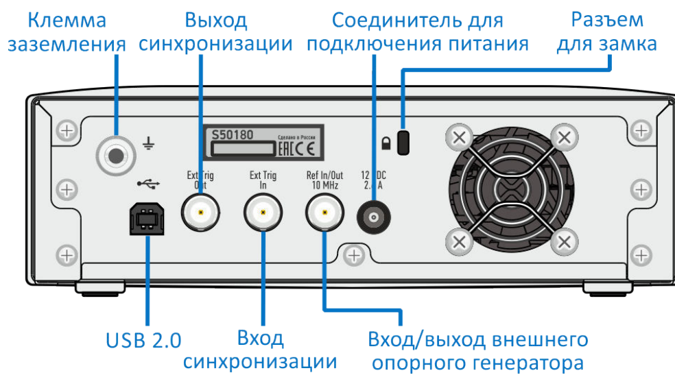
Рисунок 4.10 Задняя панель
