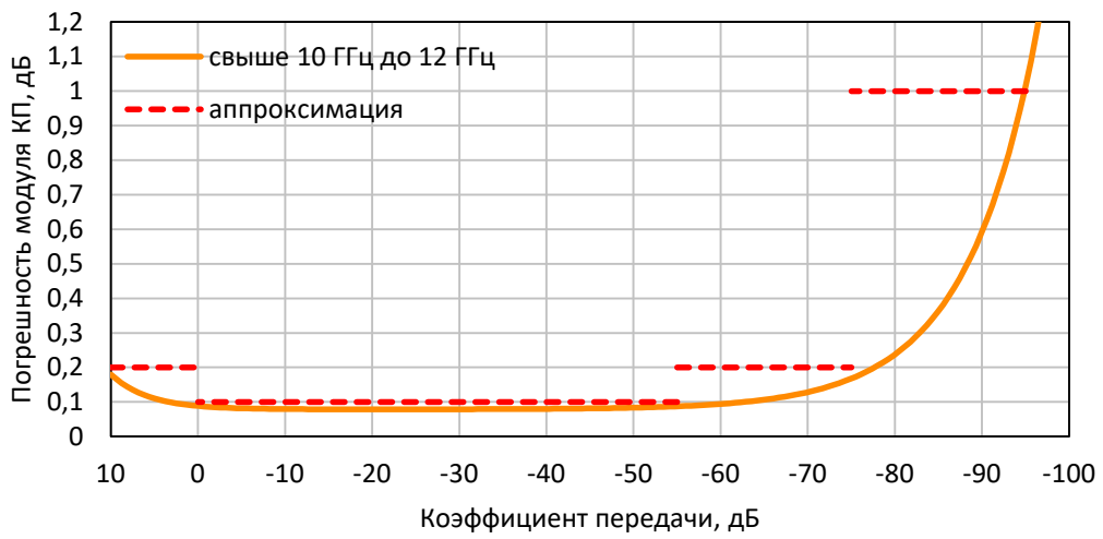
Погрешность измерений модуля коэффициента передачи согласованных устройств анализаторов S50180 (при уровне выходной мощности 0 дБм и полосе фильтра промежуточной частоты 1 Гц)
